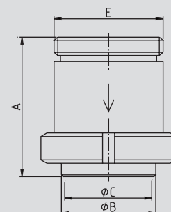
Tellerückschlagventil ZF (DIN)
