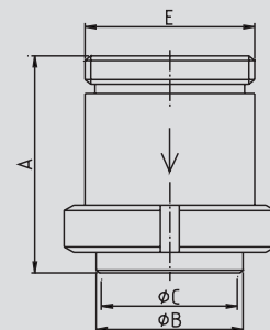
Tellerückschlagventil GS (Zoll)
